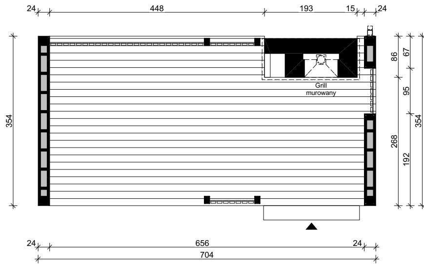
0. RZUT PARTERU
